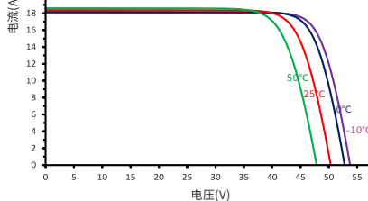
不同电池温度下, I-V 曲线图 (AM1.5, 1000W/m 2 )
